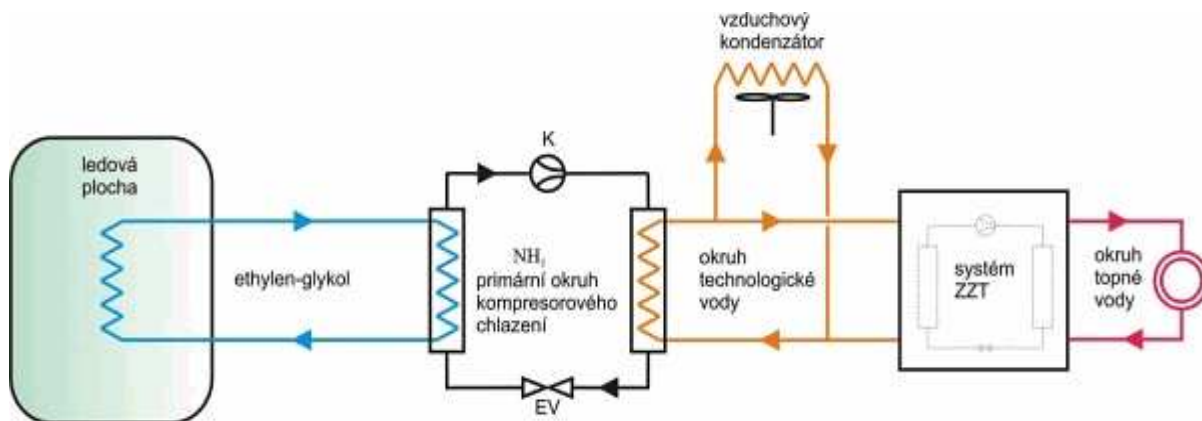
Obrázek č. 2 - Schéma systému nepřímého chlazení ledové plochy
