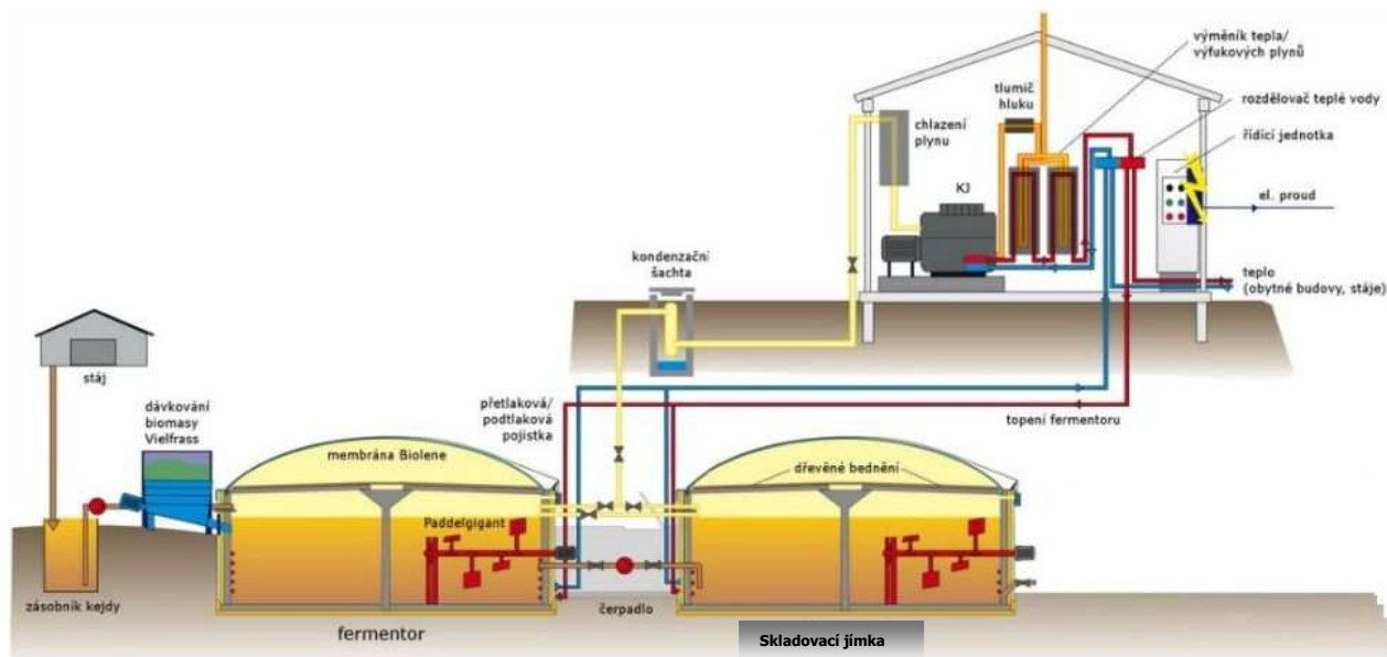
Obr.: Funkční schéma fermentační stanice
