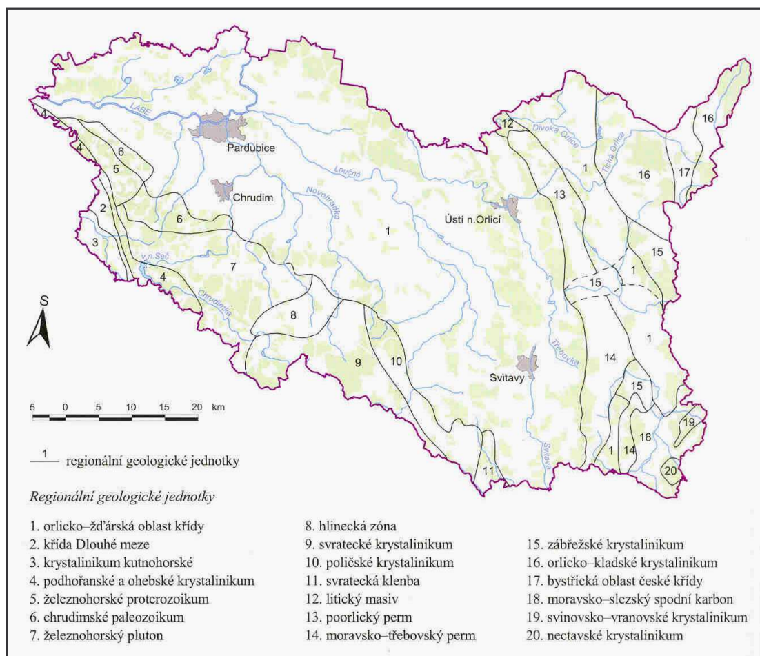
Obr. č. 6: Regionální geologické jednotky
