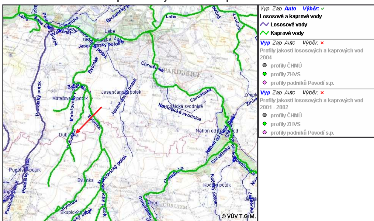
Obr. č. 7: Lososové a kaprové vody - lokalita Čepí
