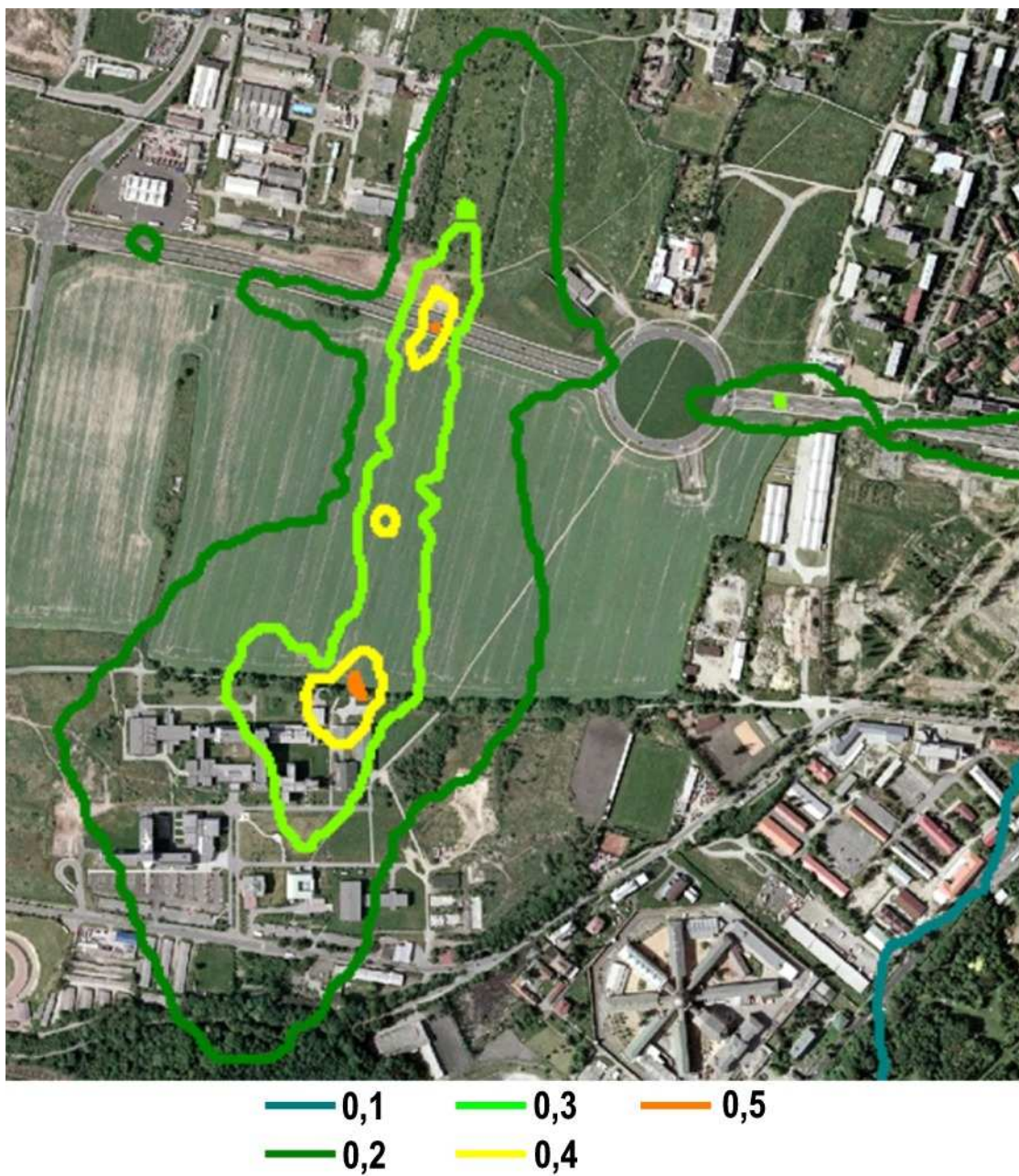
Obr.č. 5 Příspěvky maximálních hodinových imisí NO 2 (lhk) v \mu\text{g}\cdot\text{m}^{-3}
