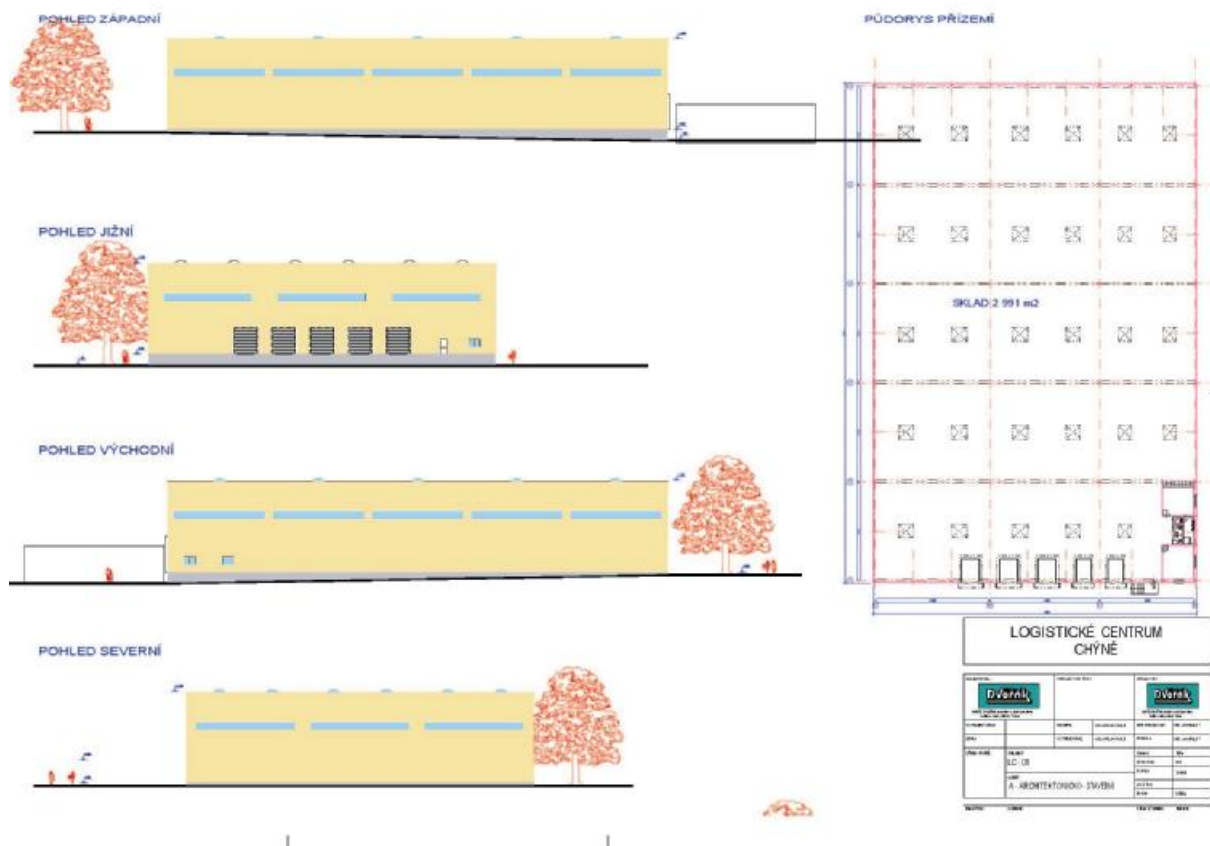
Obr. 2: Pohled na logistický objekt 1 (schéma)
