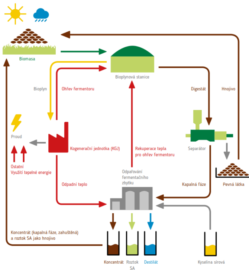
Obrázek 11: Koncepte nakládání s digestátem (zdroj www.biogastechnik-sued.com )
