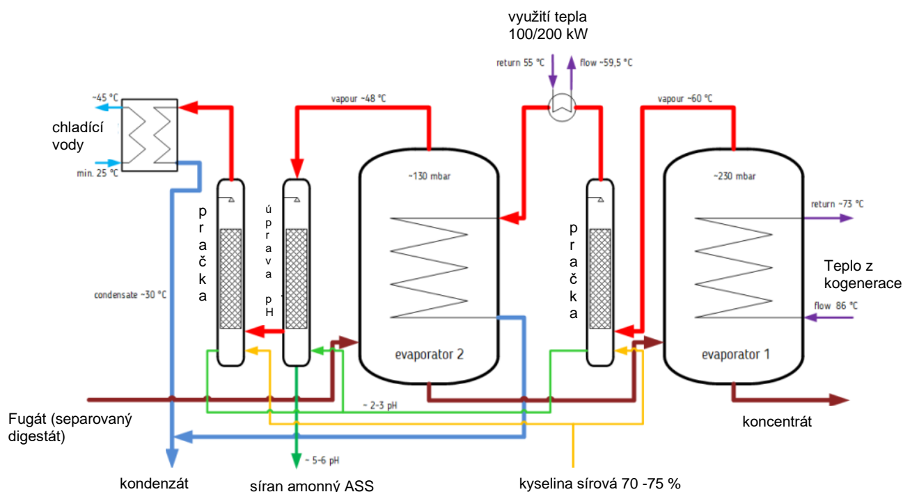
Obrázek 13: Technologické schéma evaporace digestátu (zdroj: biogastechnik-sued.com)
