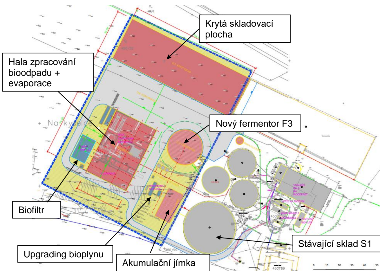
Obrázek 4: Situace umístění záměru Rozšíření bioplynové stanice Ahníkov
