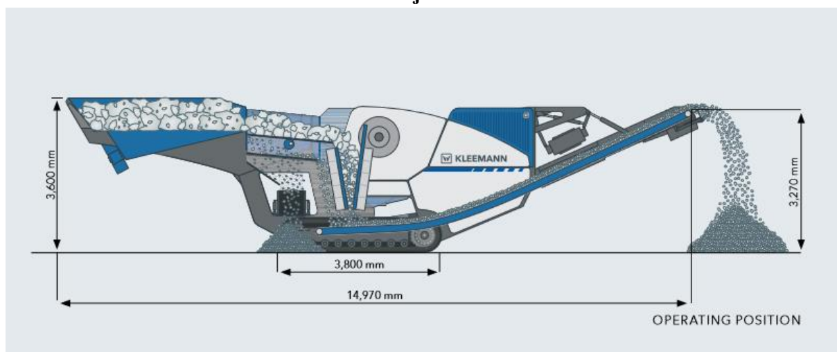
Obrázek č. 2: Nákres a popis technického řešení mobilní drtící a třídící jednotky Drťící jednotka
