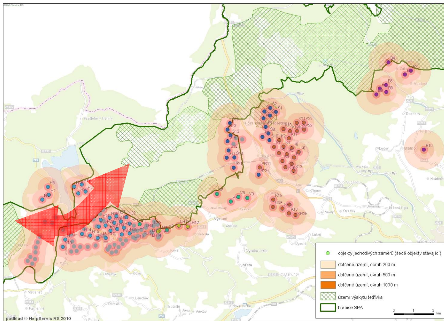
Obr. 3: Přehled všech kumulovaných záměrů v oblasti PO (= SPA) Novodomské rašeliniště - Kovářská: šedé kolečka = stávající objekty VTE + schválené VTE původního záměru Chomutov (Etapa I, II a III) a další záměry předkládané; modrá kolečka = posuzovaný záměr Větrná farma Kryštofovy Hamry a větrná farma Výsluní ; fialové kolečka + hnědá kolečka = navrhovaný záměr Větrná farma Hora Sv. Šebestiána a větrná farma Křimov; fialové kolečka = Větrná farma Blatno. Červená šipka naznačuje potenciální migrační koridor pro zachování celistvosti stávajících subpopulací tetřívka obecného ( Tetrao tetrix ) v rámci PO Novodomské rašeliniště - Kovářská.
