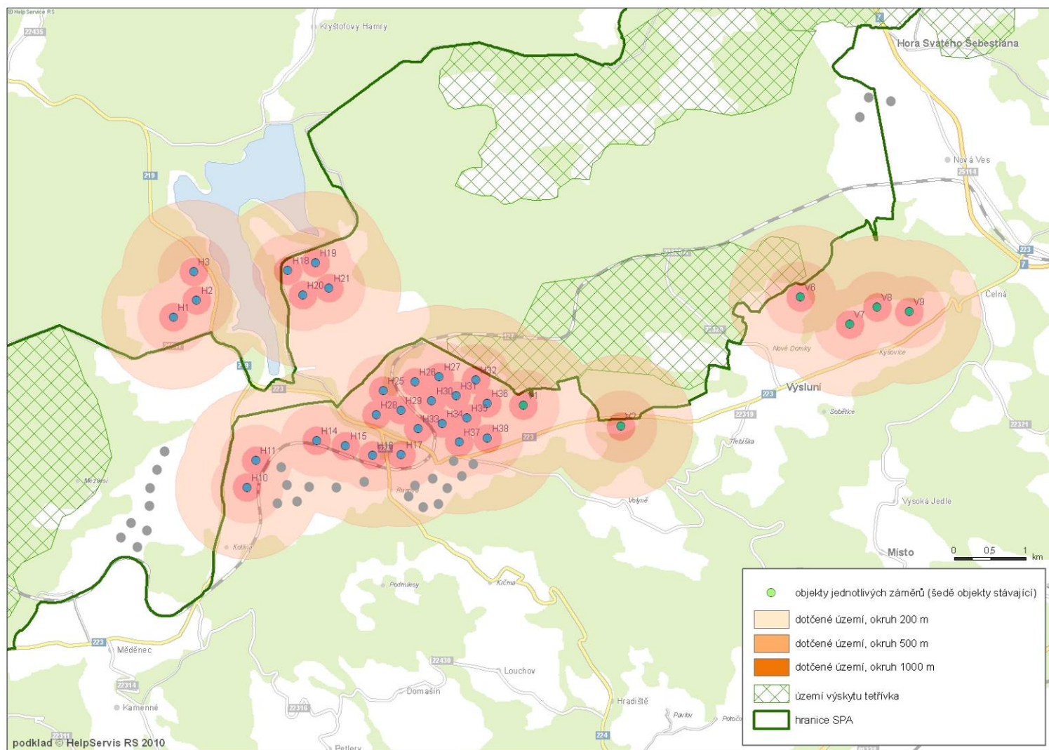
Obr. 2: Přehled navrhovaných VTE v rámci záměru "Větrná farma Kryštofovy Hamry a větrná farma Výsluní", s vyznačením zón překryvu s místy výskytu tetřívka obecného ( Tetrao tetrix ).
