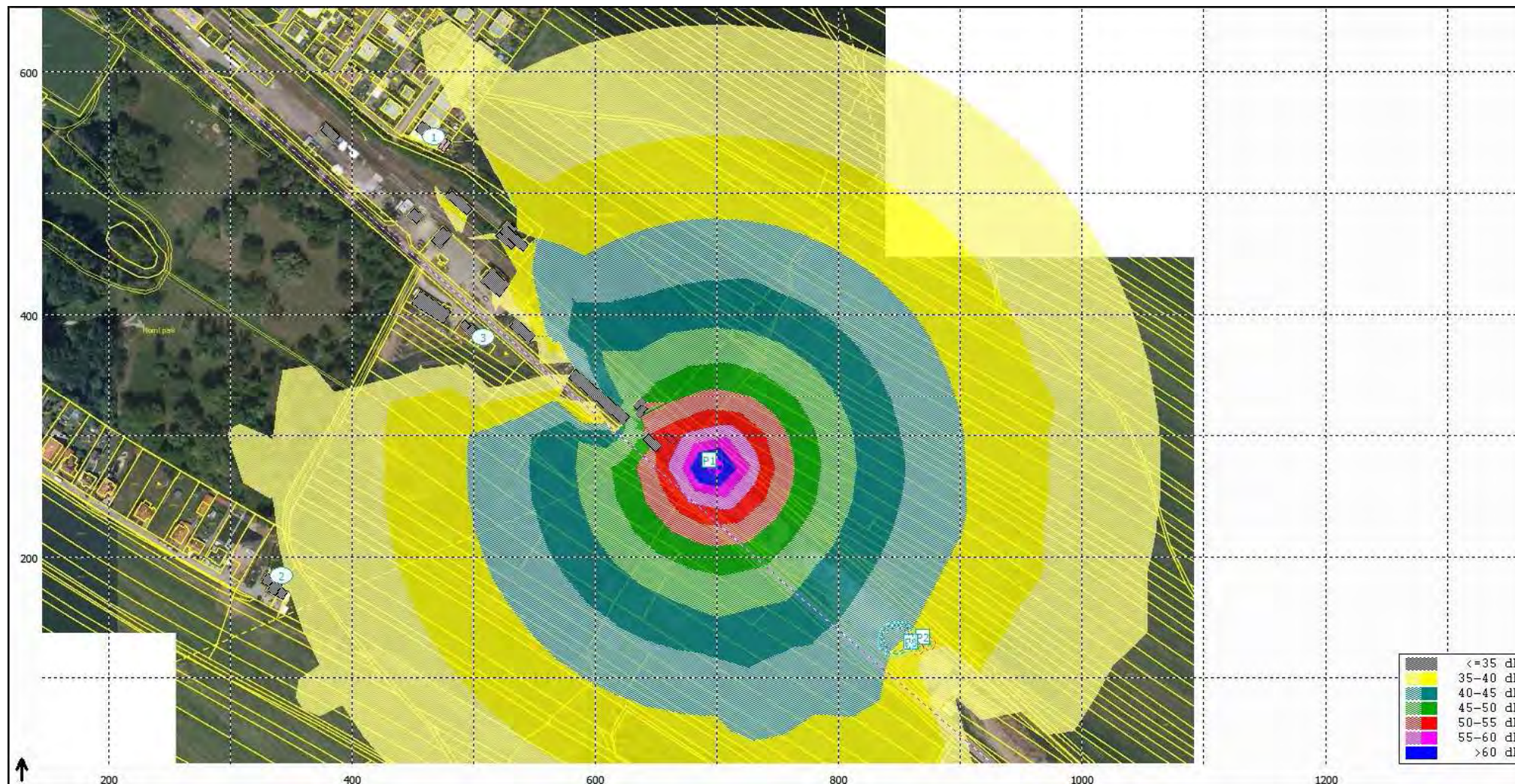
OBR. 2 Hladiny ak. tlaku A ve výšce 3 m nad terénem, stávající hluková situace – stacionární zdroje OPAMETAL s. r. o.
