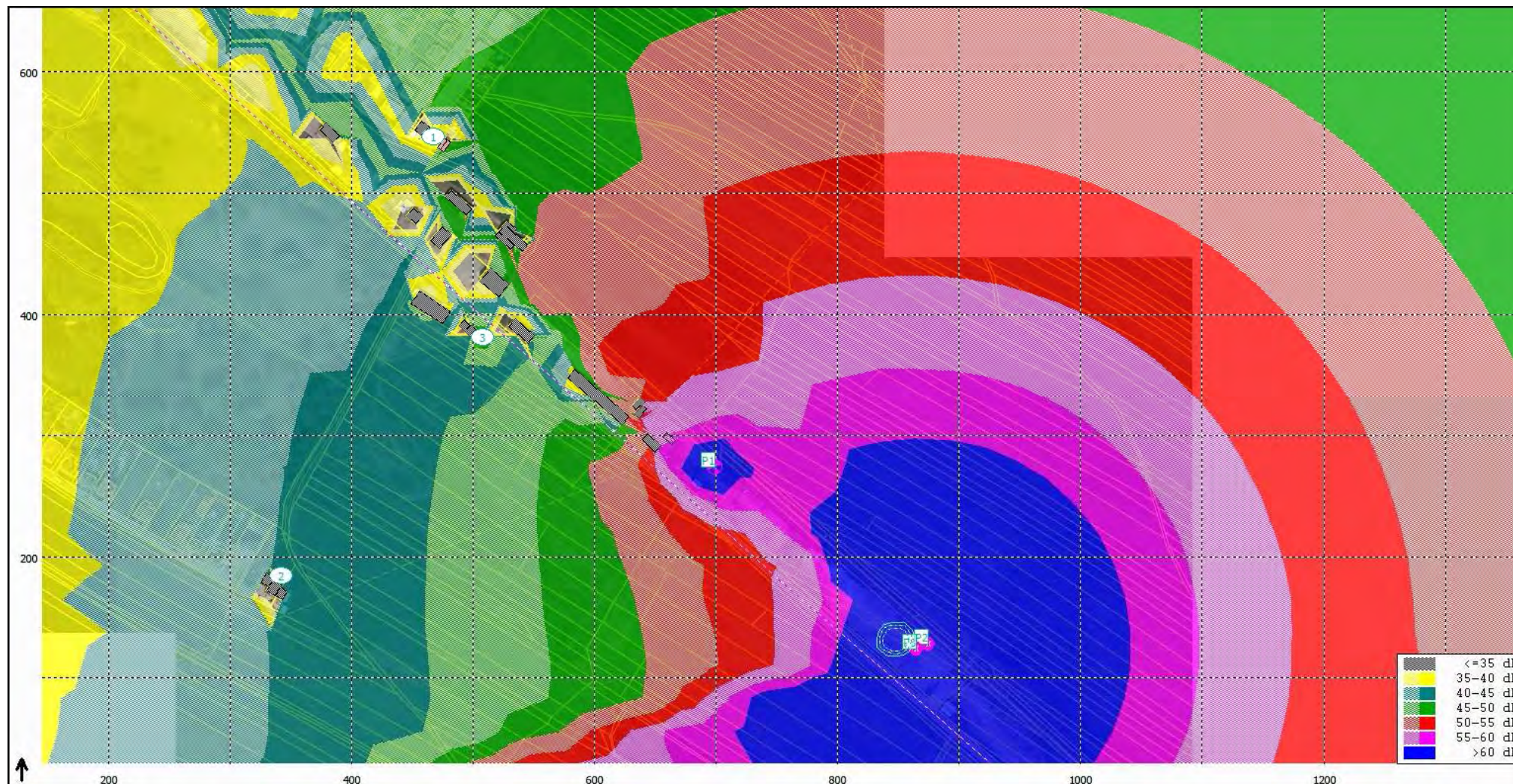
OBR. 3 Hladiny ak. tlaku A ve výšce 3 m nad terénem, výhledová hluková situace – stacionární zdroje ČECH-ODPADY s.r.o.
