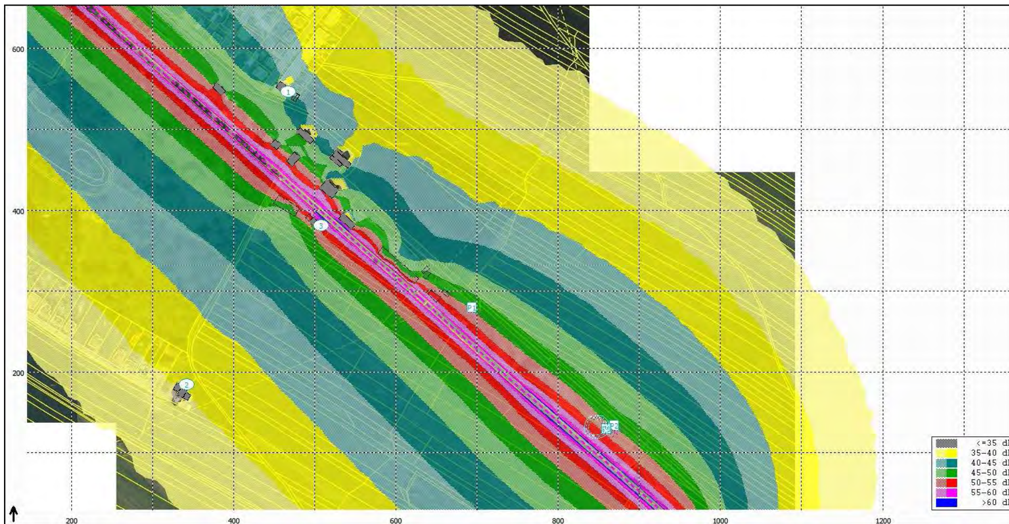
OBR. 1 Hladiny ak. tlaku A ve výšce 3 m nad terénem, stávající hluková situace – doprava po silnici II/408
