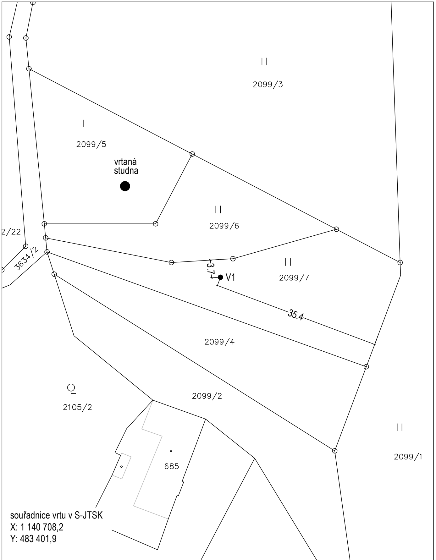
Obr. 2 Katastrální situační výkres v měřítku 1 : 500
