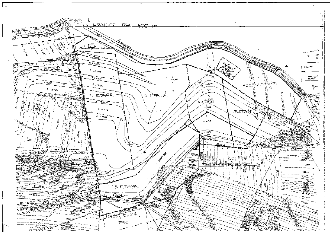
Obrázek 1: situační plánec biokoridoru a 5. etapy skládky (podklad obce Těmice)
