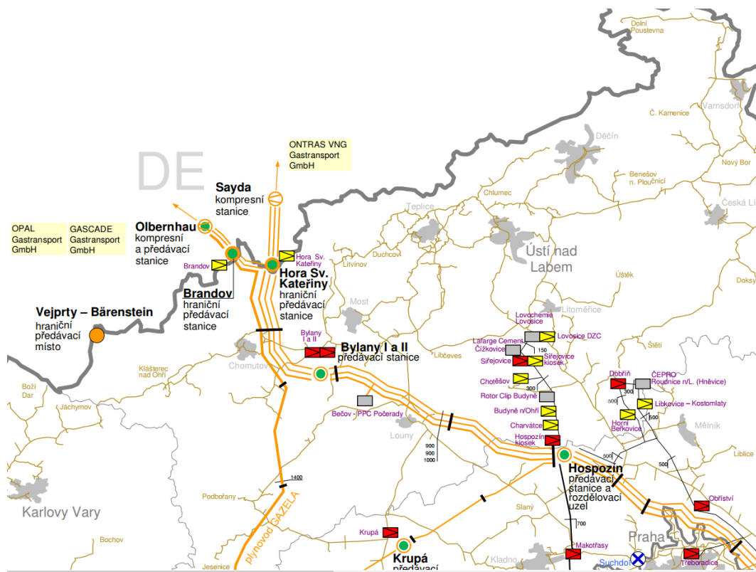
Obr. 41 Soustava zásobování kraje zemním plynem, 2016
