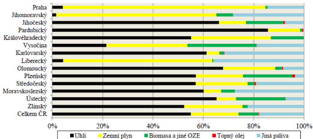
Obr. 27 Druhy paliv použitých pro výrobu tepelné energie za rok 2016 po jednotlivých krajích
