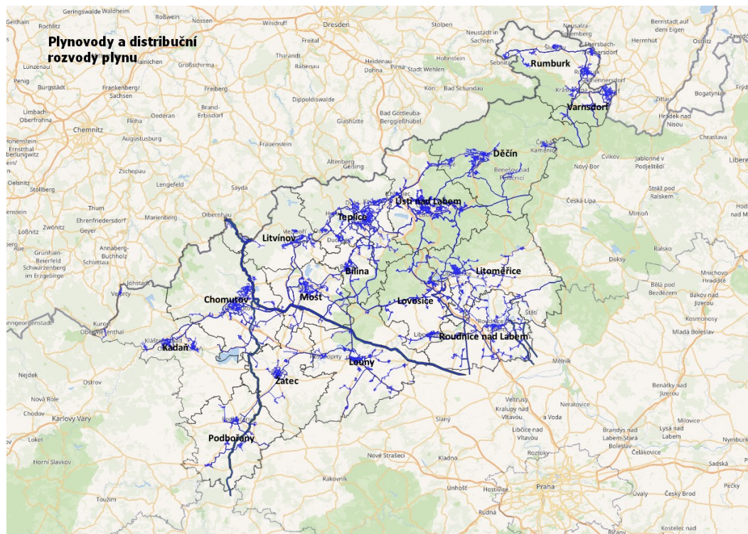
Obr. 42 Plynovody a distribuční rozvody plynu
