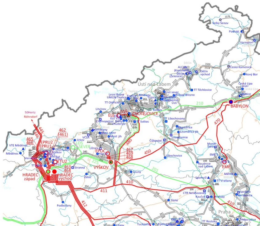
Obr. 39 Elektrizáční soustava Ústeckého kraje v roce 2015
