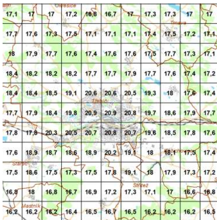
Obrázek 7: Území města Třebíč, PM 10 – pětiletý průměr roční koncentrace, 2016-2020 (zdroj: https://chmi.cz/ ) Limit 40 µg/m 3 není překračován.
