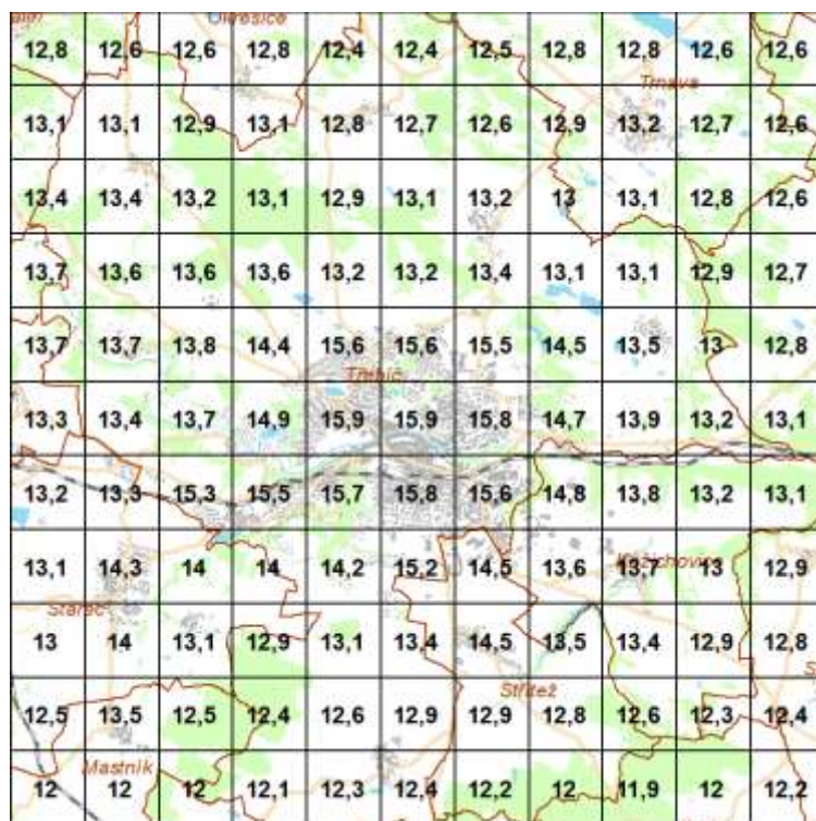
Obrázek 8: Území města Třebíč, PM 2,5 – pětiletý průměr roční koncentrace, 2016-2020 (zdroj: https://chmi.cz/ ) Imisní limit 20 µg/m 3 není překračován ani v místech s vyšší intenzitou dopravy.
